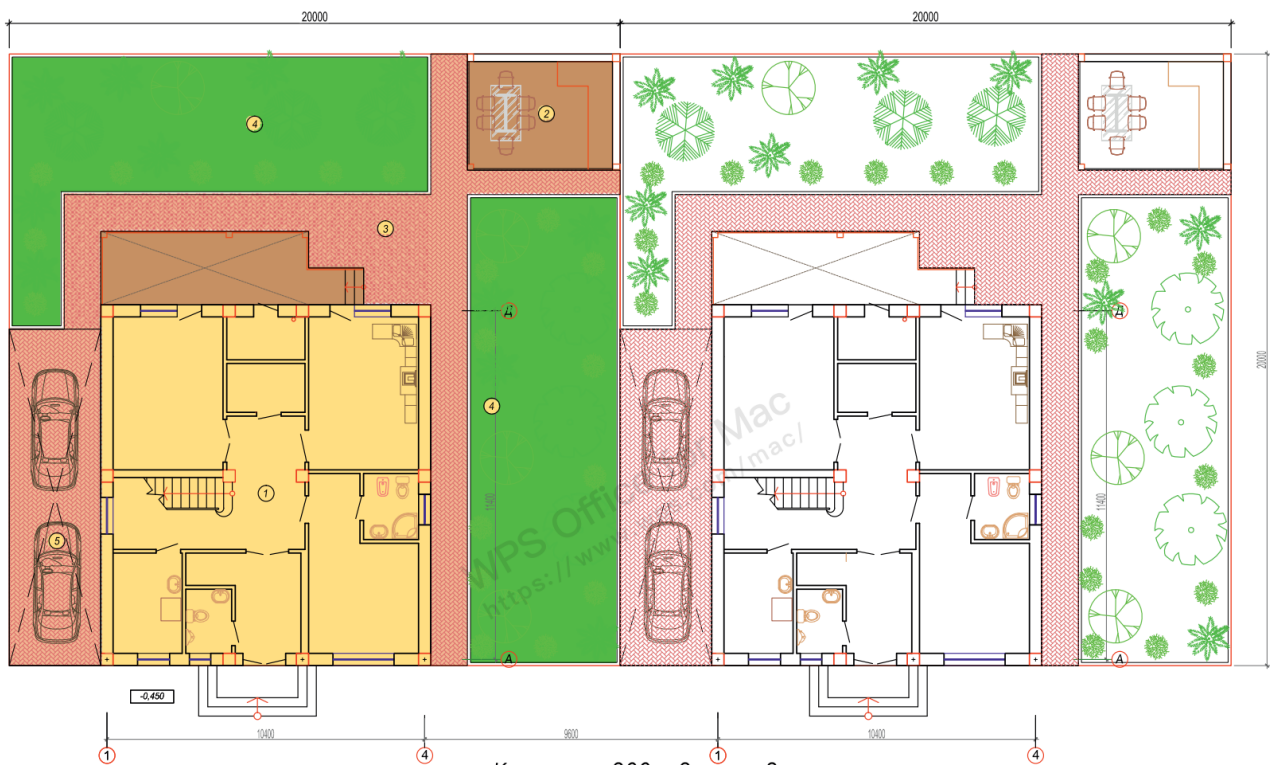
Коттедж - 200 м2 тип - 2
